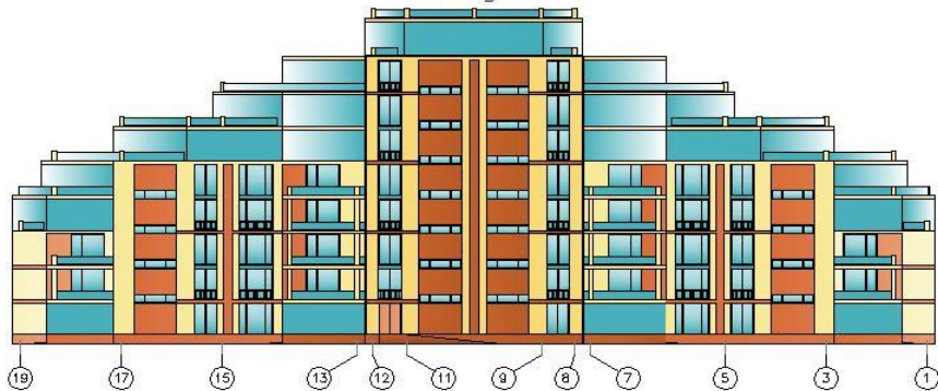
Фасад 19-1
