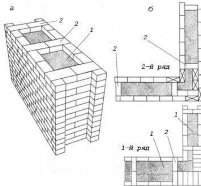
Рис. 5. «Колодцевая» кладка: а- фрагмент кладки; б- порядковая раскладка кирпичей при кладке прямого угла стены; 1- утеплитель; 2- диафрагма из тычковых кирпичей.
