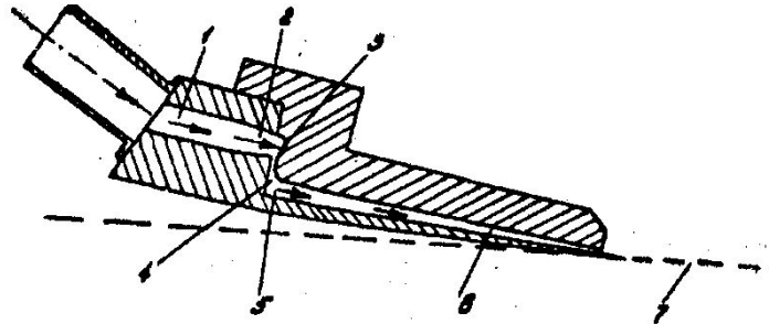
Рис. 62. Принципиальная схема формования полотна методом экструзии: 1-2-3-4-5-6 - экструзионные зоны; 7 - сетка.
