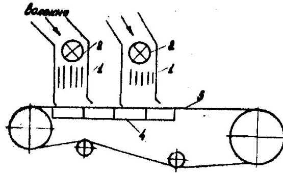
Рис. 61. Принципиальная схема двухважной машины для сухого формования: 1 - шакта; 2 - питатель; 3 - бесконечная сетка; 4 - формирующее устройство.
