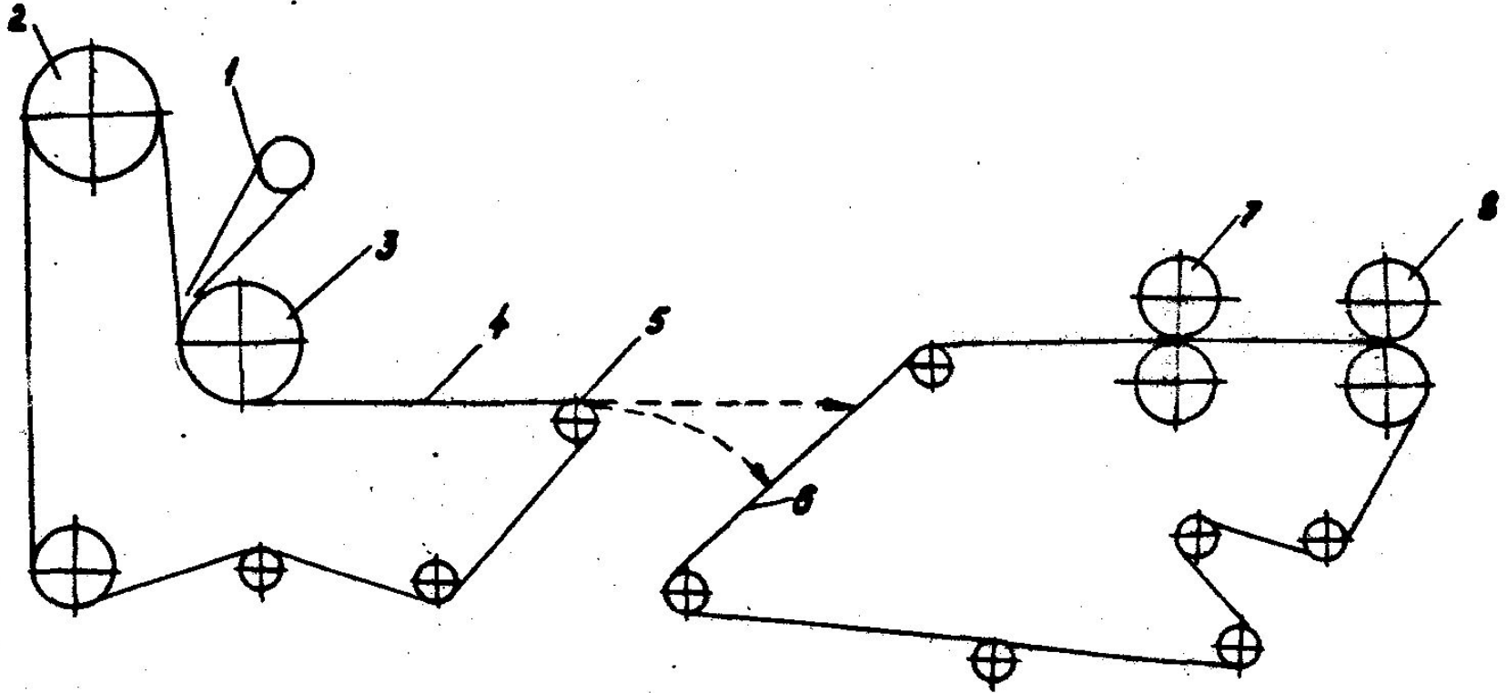
Рис. 59. Схема машины «Кивач» с отдельным формованием и обезвоживанием бумажного полотна:
