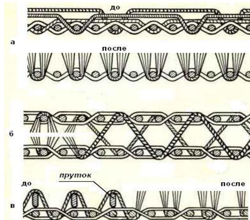
Ворсовые переплетения (разрезы)
