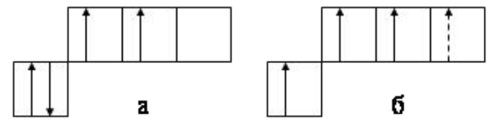
Рис.2 Электронное строение атома углерода и его внешнего электронного слоя с валентностью равной: а) двум, б) четырем
