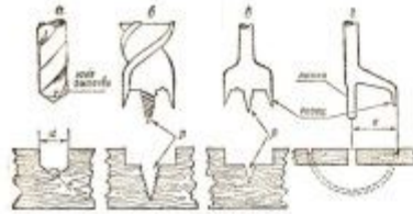
Трассы, образованные режущей кромкой сверла, на дне следа сверления.
