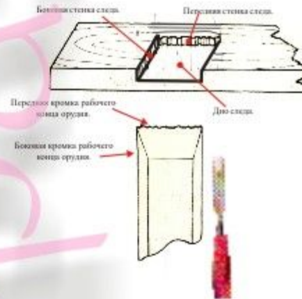
Объемный (вдавленный) след, образованный рабочим концом ломика.
