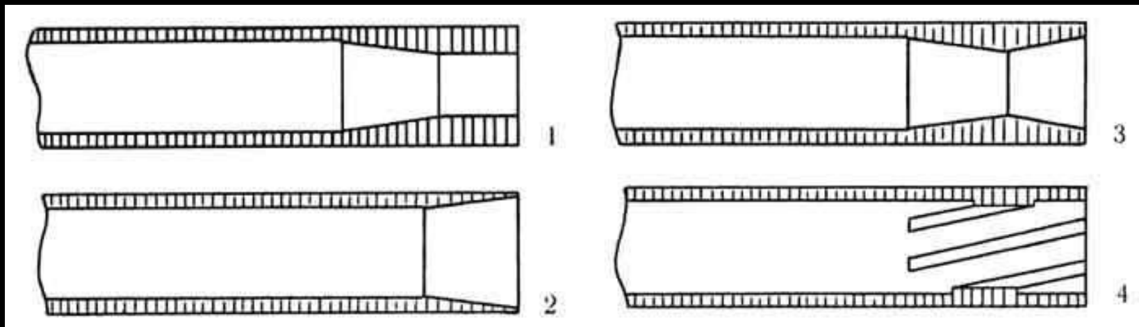
Виды сверловки канала ствола гладкоствольного оружия
