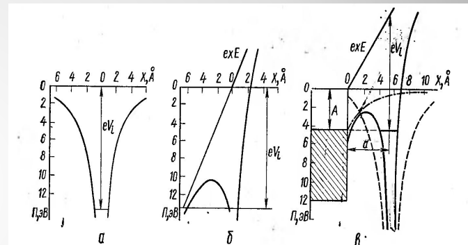
Рис. 9.14. Потенциальные диаграммы свободного атома: а — без поля; б — в электрическом поле; в — в электрическом поле вблизи металлической поверхности
