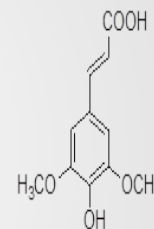
Синаповая (гидрокси метокси коричная) кислота, SA
