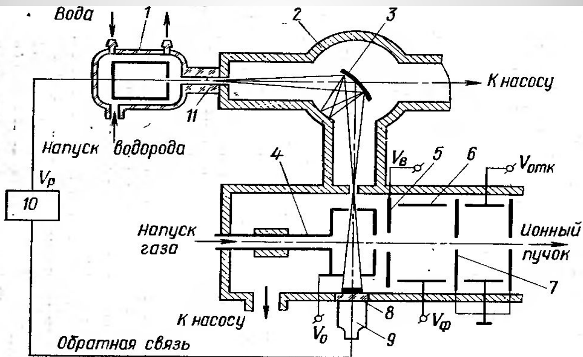
Рис. 9.12. Схема фотоионизационного источника:
