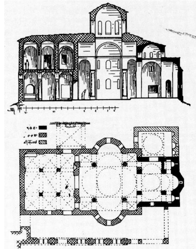
Розріз та план Преображенського Собору
