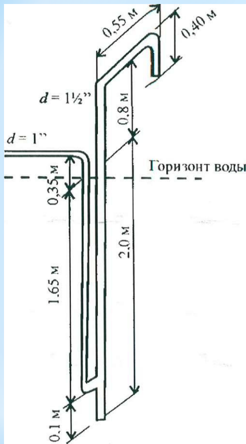
Схема контрольного эрлифта вторичного отстойника
