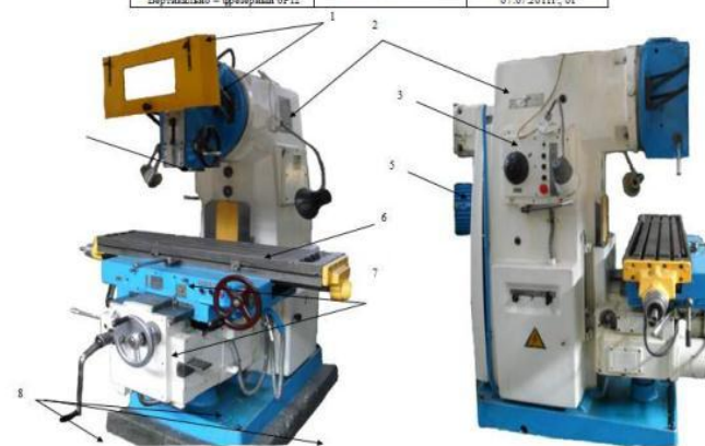
План чистки вертикально-фрезерного станка 6P12.
