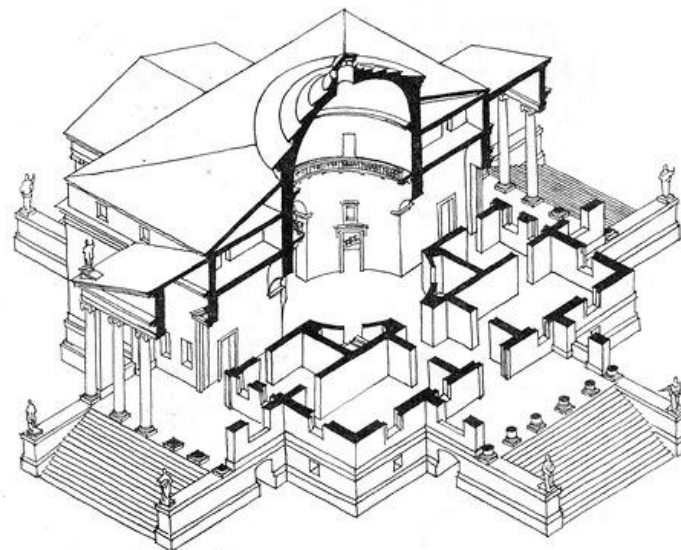
Вилла Ротонда. Палладио. 1566 г.
