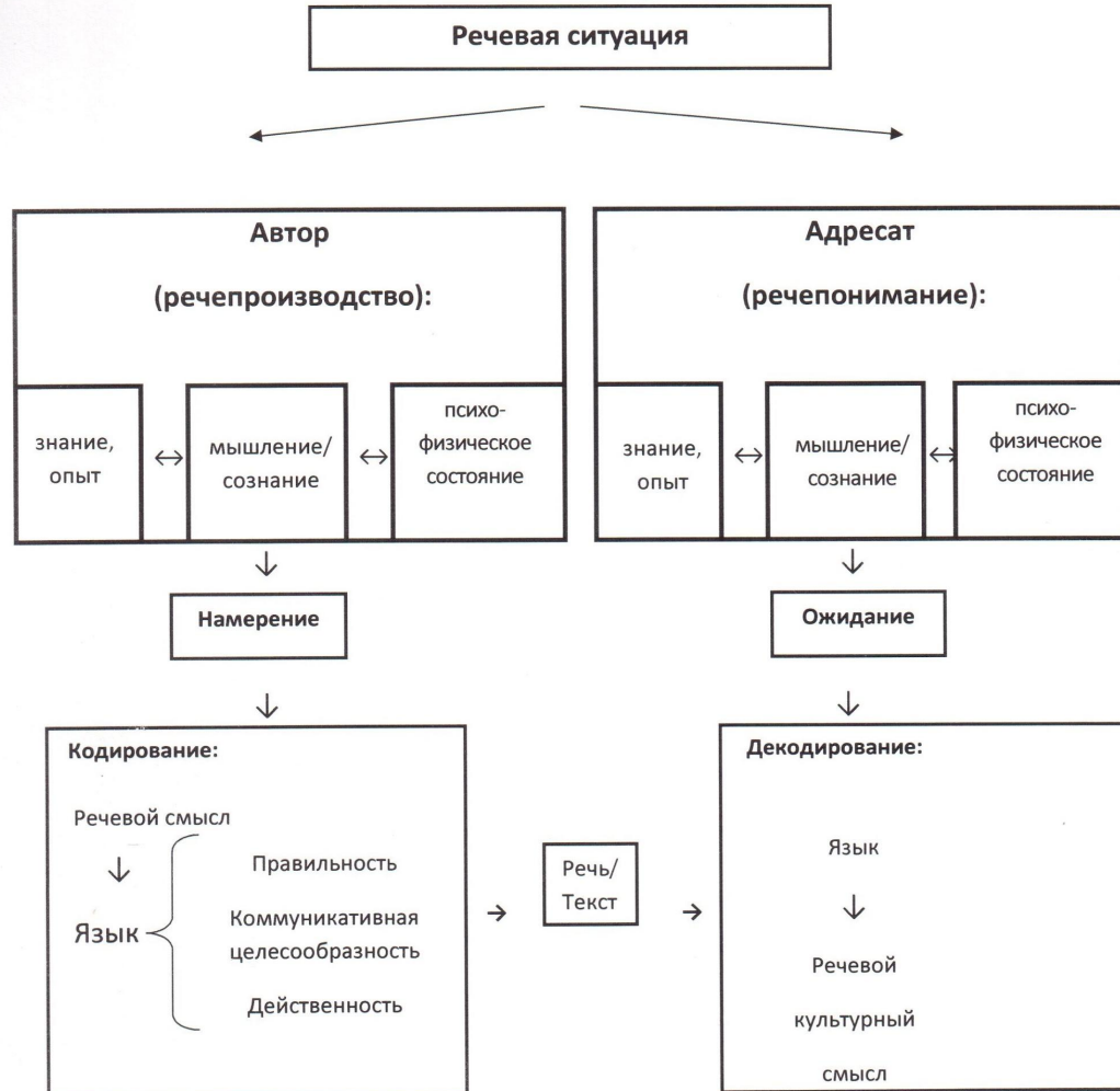
Графическая модель коммуникативного акта
