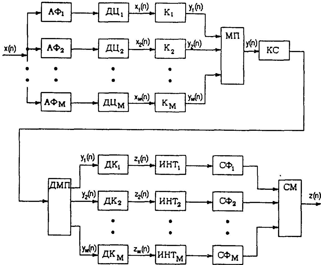
Рис. 3.2 Структурная схема системы передачи сигнала с разложением на частотные поддиапазоны
