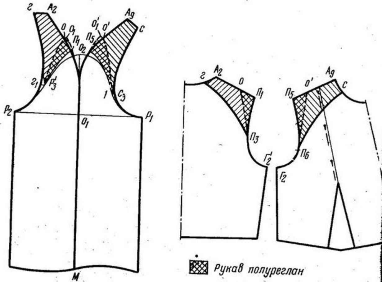
Рис. 24. Чертеж лифа платья покроя реглан, построенный на лекалах лифа платья с втачными рукавами
