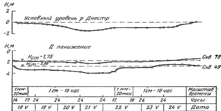
Рис. Графіки коливанні рівнів у спостережних свердловинах при дослідній відкачці з куща 55 під впливом зміни рівня в ріці (за даними Л. П. Шараєвського, 1970р. долина р. Дністер)
