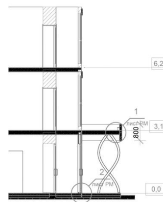
РАЗРЕЗ 1-1
