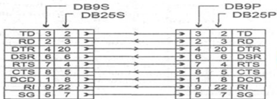
Кабели подключения модемов
