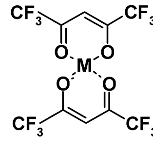
M(hfac) 2
