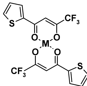
M(tta) 2
