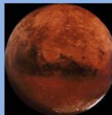
Марс
