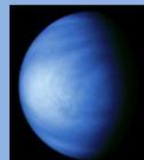
Венера
