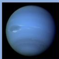
Нептун
