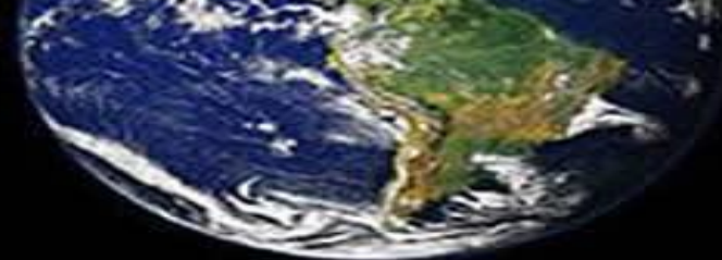
Земля
