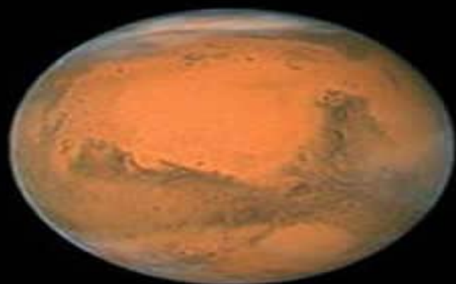
Марс
