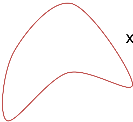
замкнутая кривая
