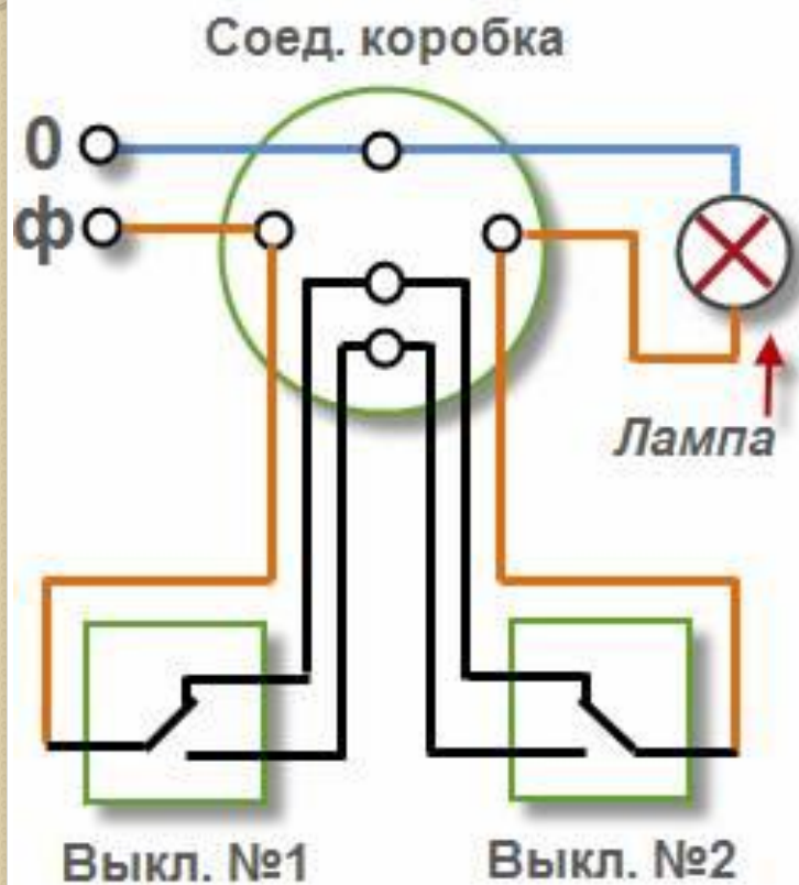
Схема управления светильником из 2 мест.
