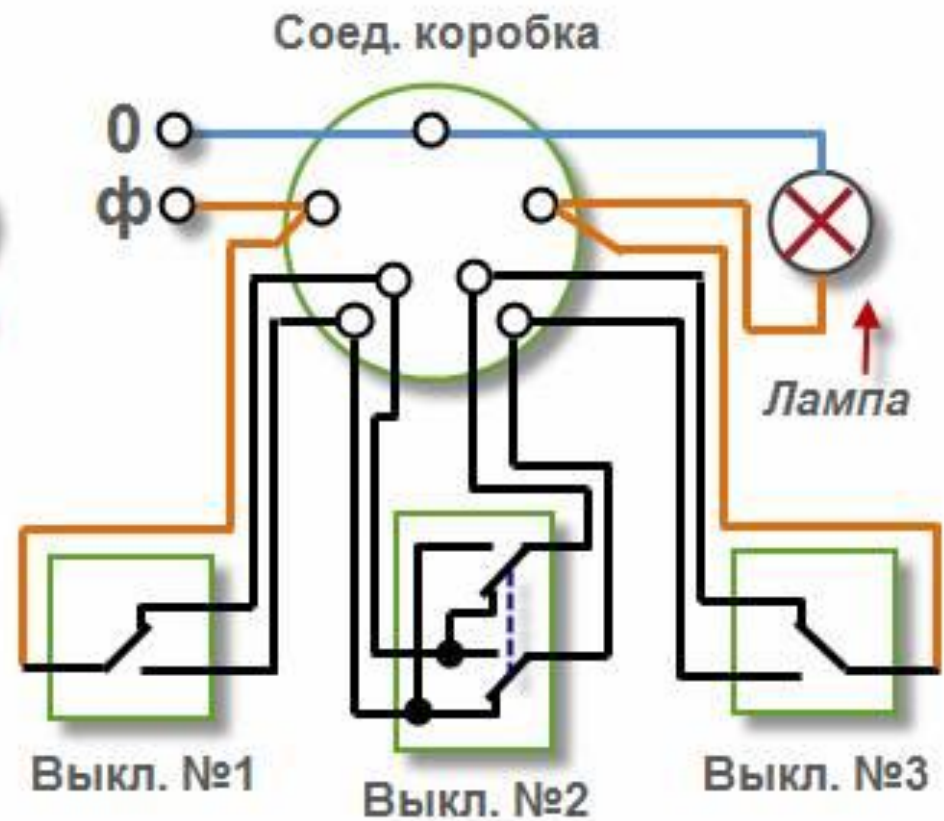
Схема управления светильником из 3 мест.
