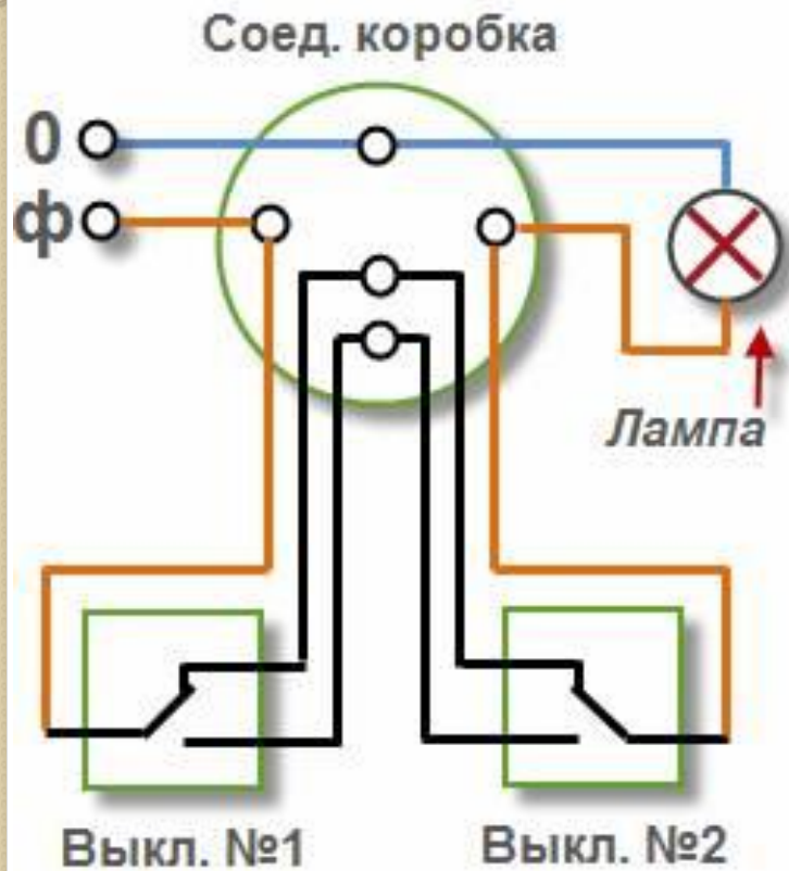
Схема управления светильником из 2 мест.
