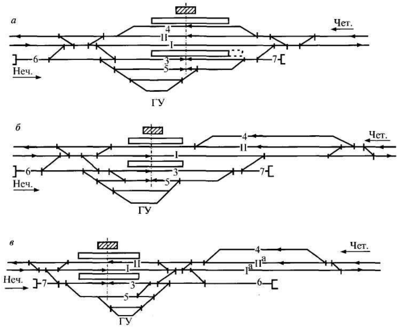
Рис. 3.7. Схемы промежуточных станций на двухпутной линии с расположением путей: a — поперечным; б — полупродольным; в — продольным
