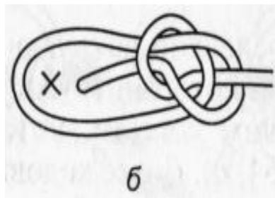
«Булинь»
