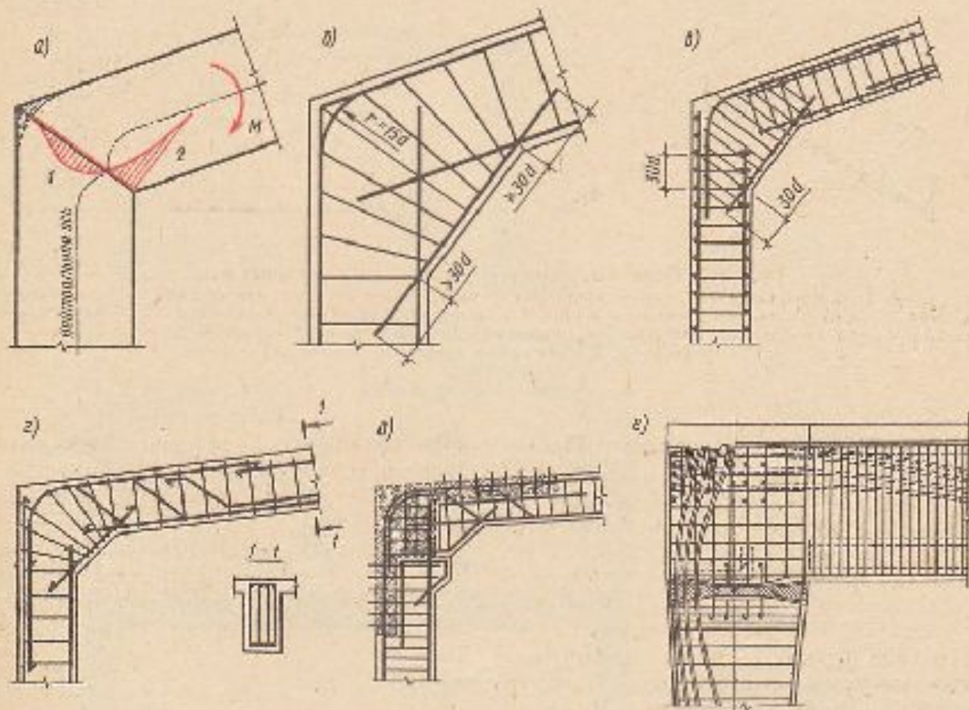
Рис. 5.71. Карнизные узлы железобетонных рам:
