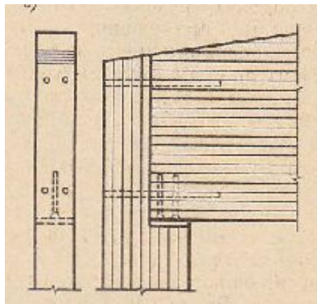
- на клеенных штырях
