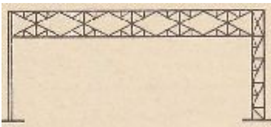
В) ... с гибкой и жесткой стойками
