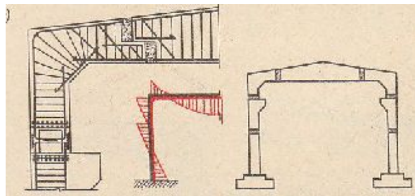
бесшарнирная из 7-и элементов
