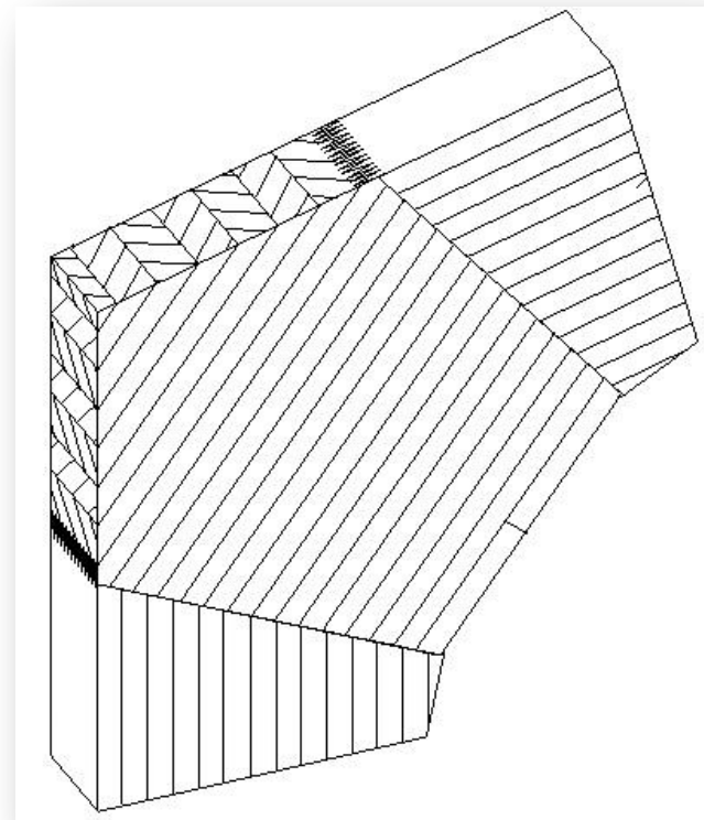
Рис. 9 Соединение ригеля и стойки при помощи пятиугольной вставки
