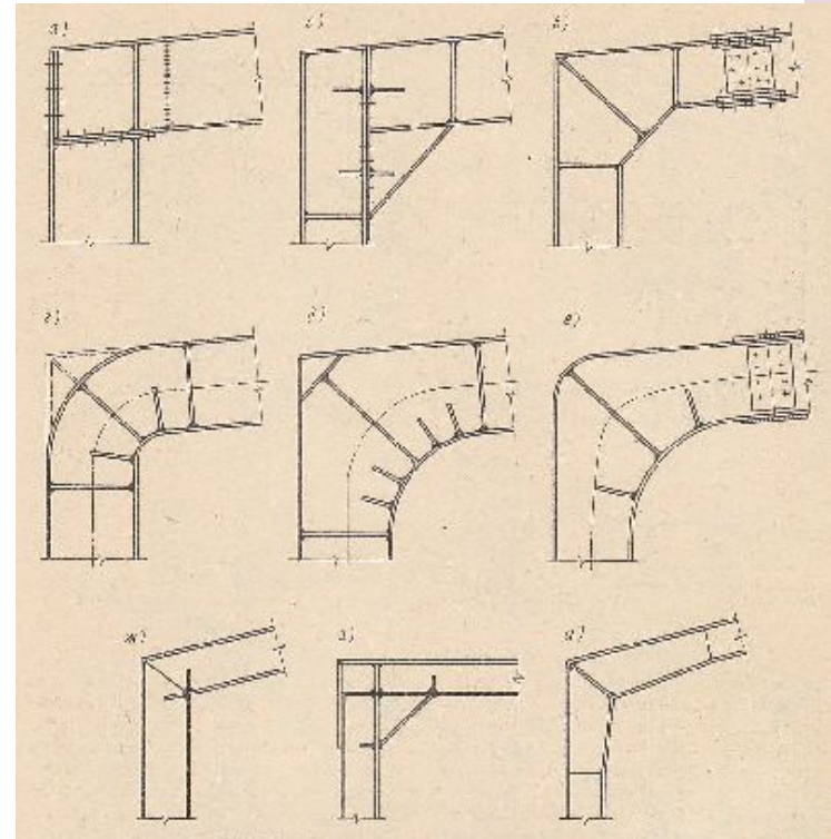
Карнизные узлы сплошнотенчатых стальных рам
