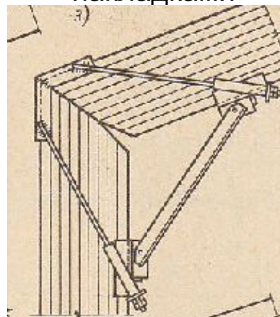
- со стальным хомутом
