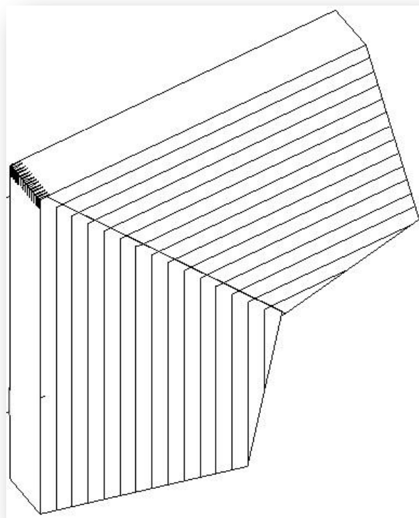
Рис. 8 Соединение ригеля со стойкой на зубчатый шип
