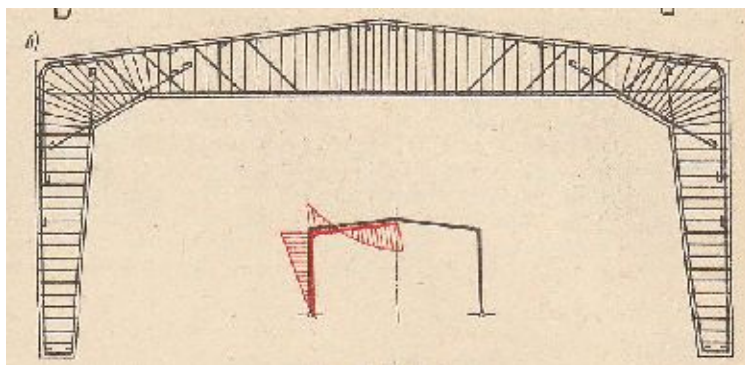
двухшарнирная монолитная
