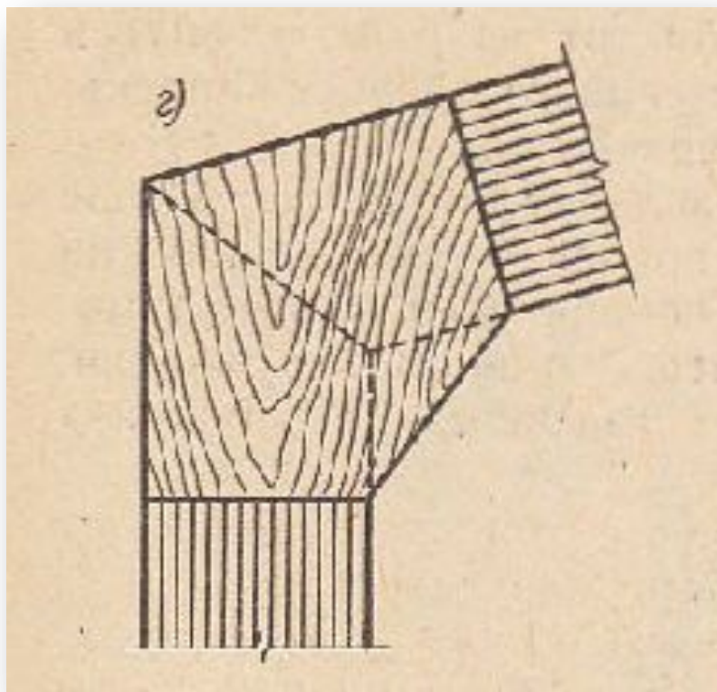
Рис. 7 Соединение ригеля и стойки накладками из фанеры
