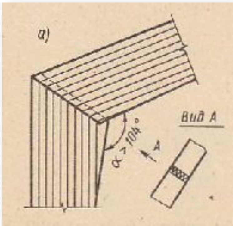
Рис. 8 Соединение ригеля со стойкой на зубчатый шип
