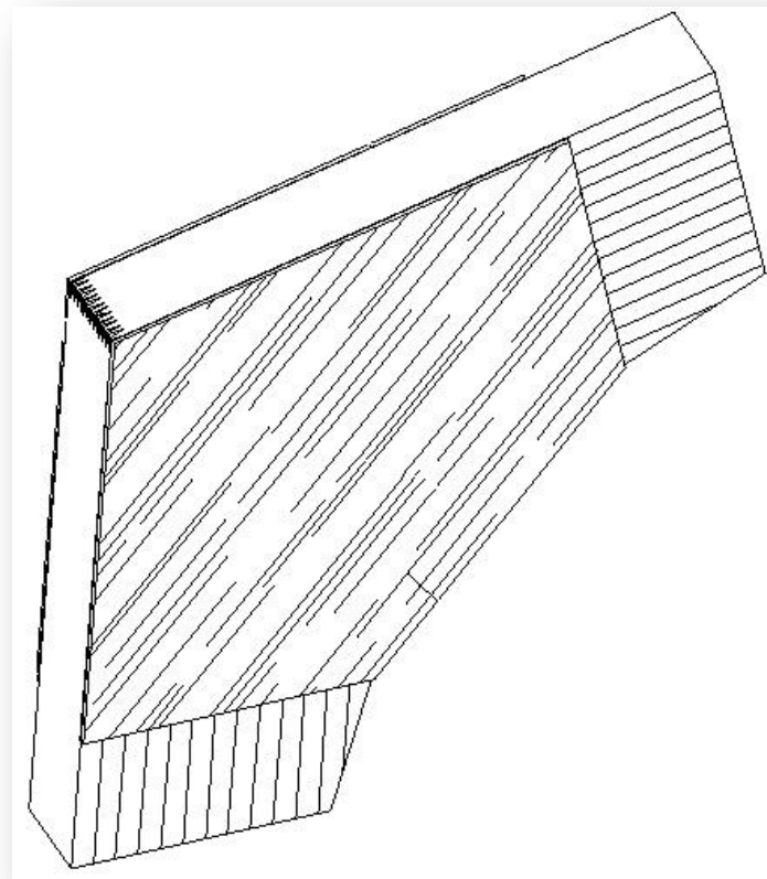
Рис. 7 Соединение ригеля и стойки накладками из фанеры
