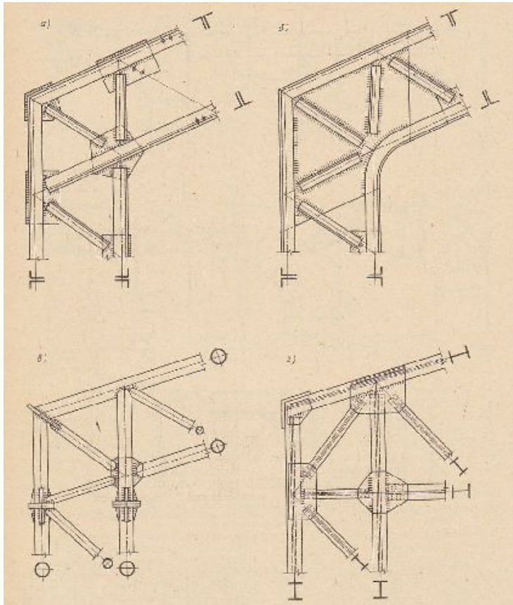
Карнизные узлы сквозных рам
