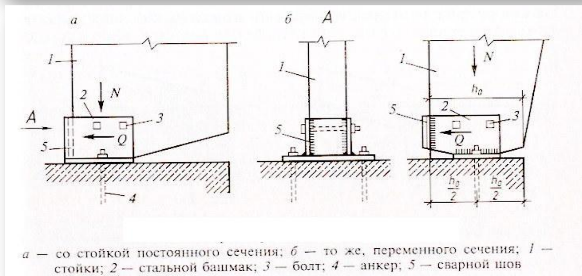
Рис. 18 Варианты опорных узлов
