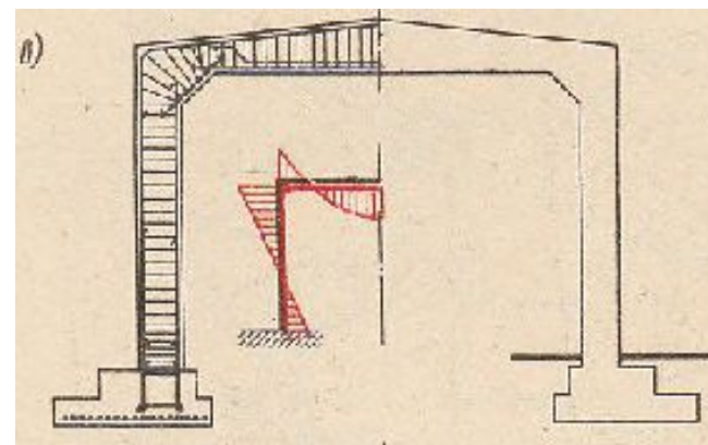
бесшарнирная монолитная
