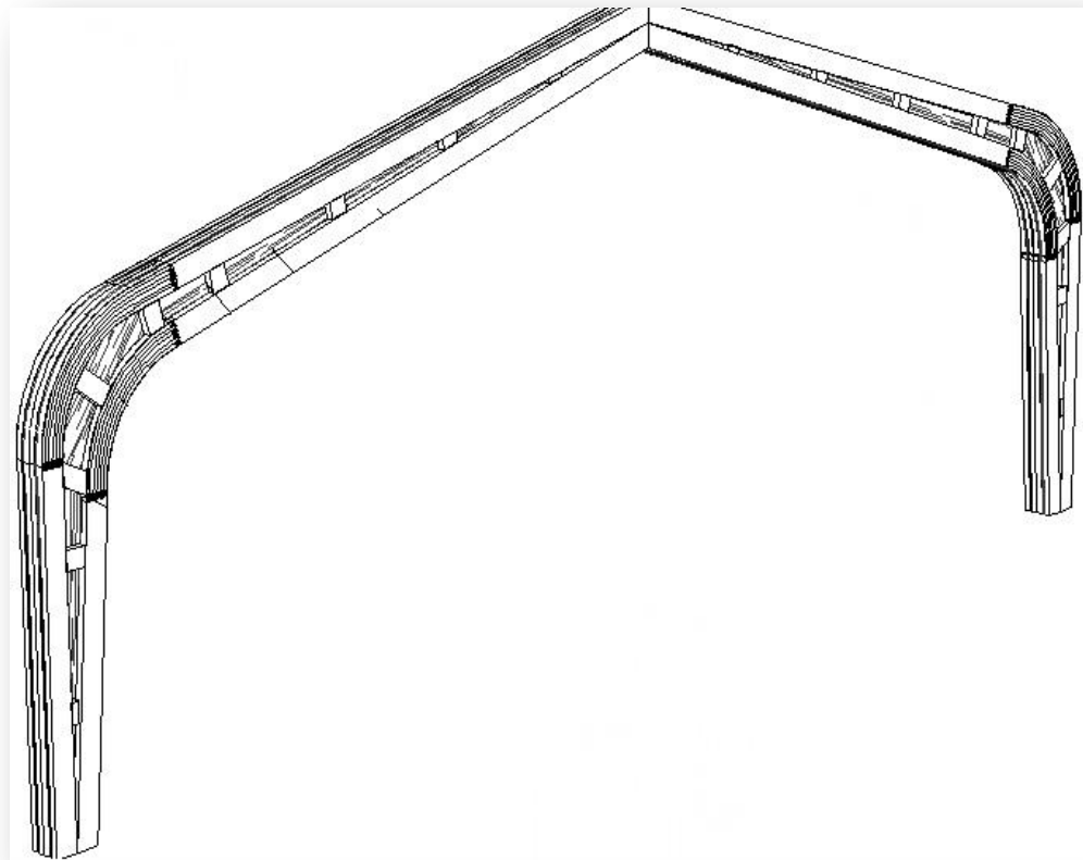
Рис. 12 Клеифанерная рама
