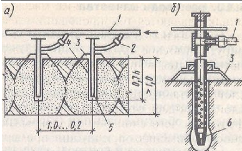
Рис. 26. Оттаивание грунта паром (размеры в м): a – общая схема; б – паровая игла; 1 – паропровод; 2 – паровой вентиль; 3 – колпак; 4 – пробуренная скважина; 5 – паровая игла; 6 – наконечник
