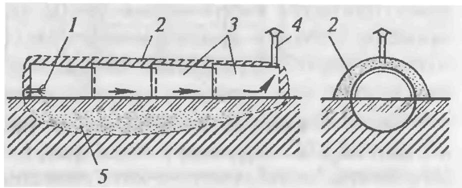
Рис. 22. Установка для оттаивания грунта жидким топливом:
