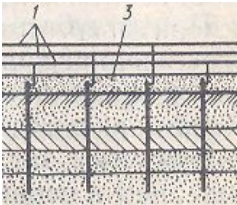
Рис. 25. Оттаивание грунта способом электропрогрева вертикальными электродами сверху вниз и снизу вверх (размеры в м):
