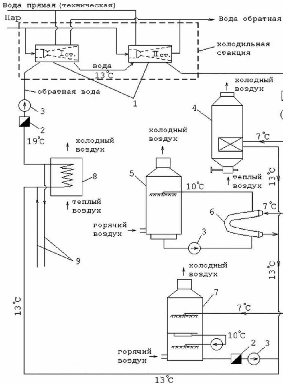
Принципиальная схема холодоснабжения металлургического завода (пароэжекторный способ получения холода)
