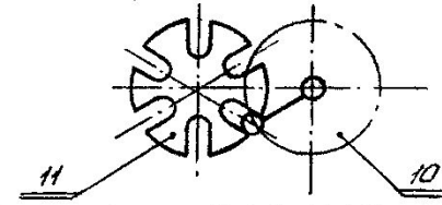
Вид сверху на механизм с мальтийским крестом (наружное зацепление)
