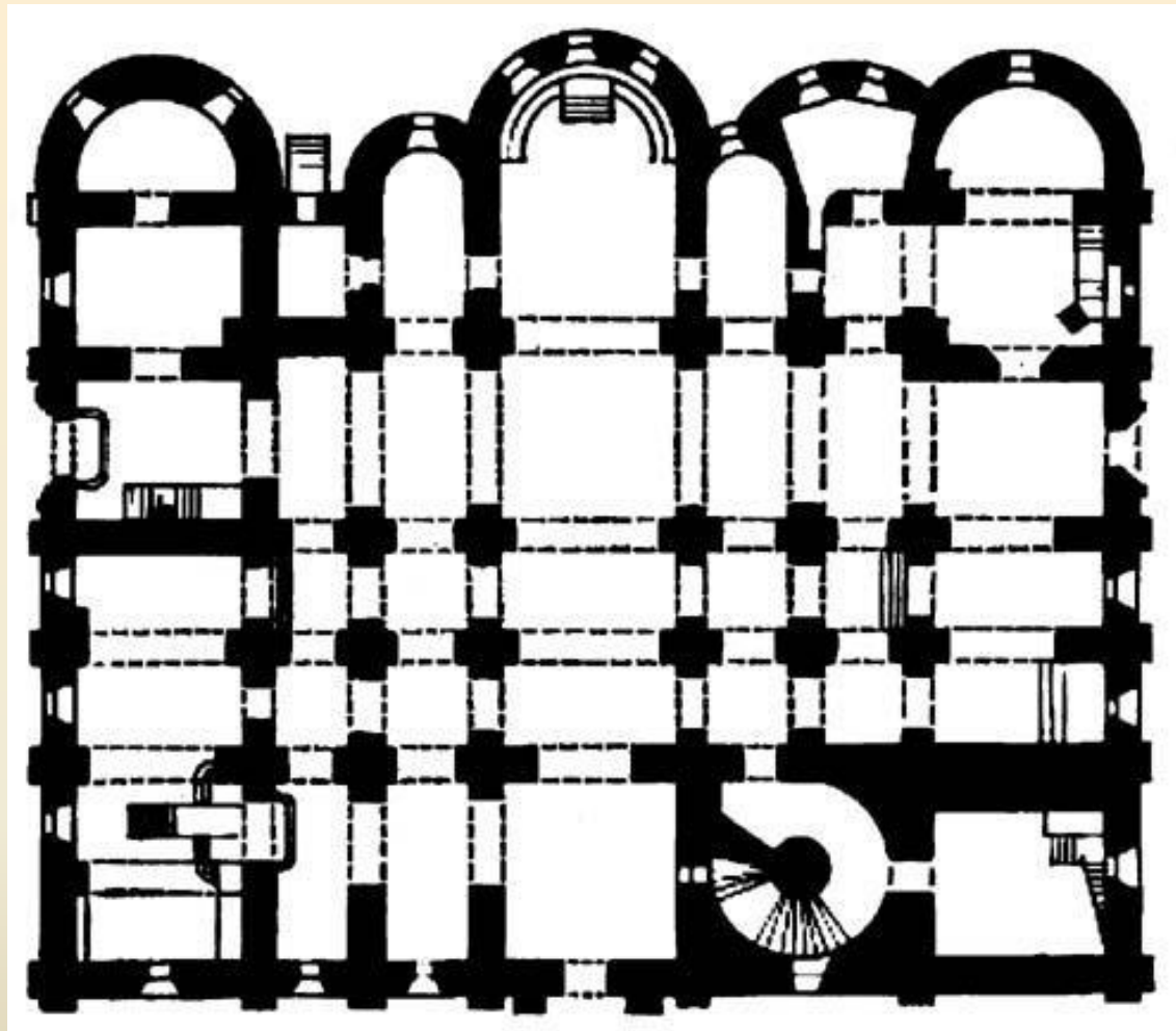
План собора Святой Софии в Новгороде
