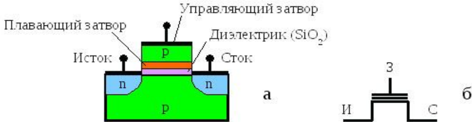
Структура полевого транзистора с плавающим затвором (а) и его обозначение на электрических схемах (б).
