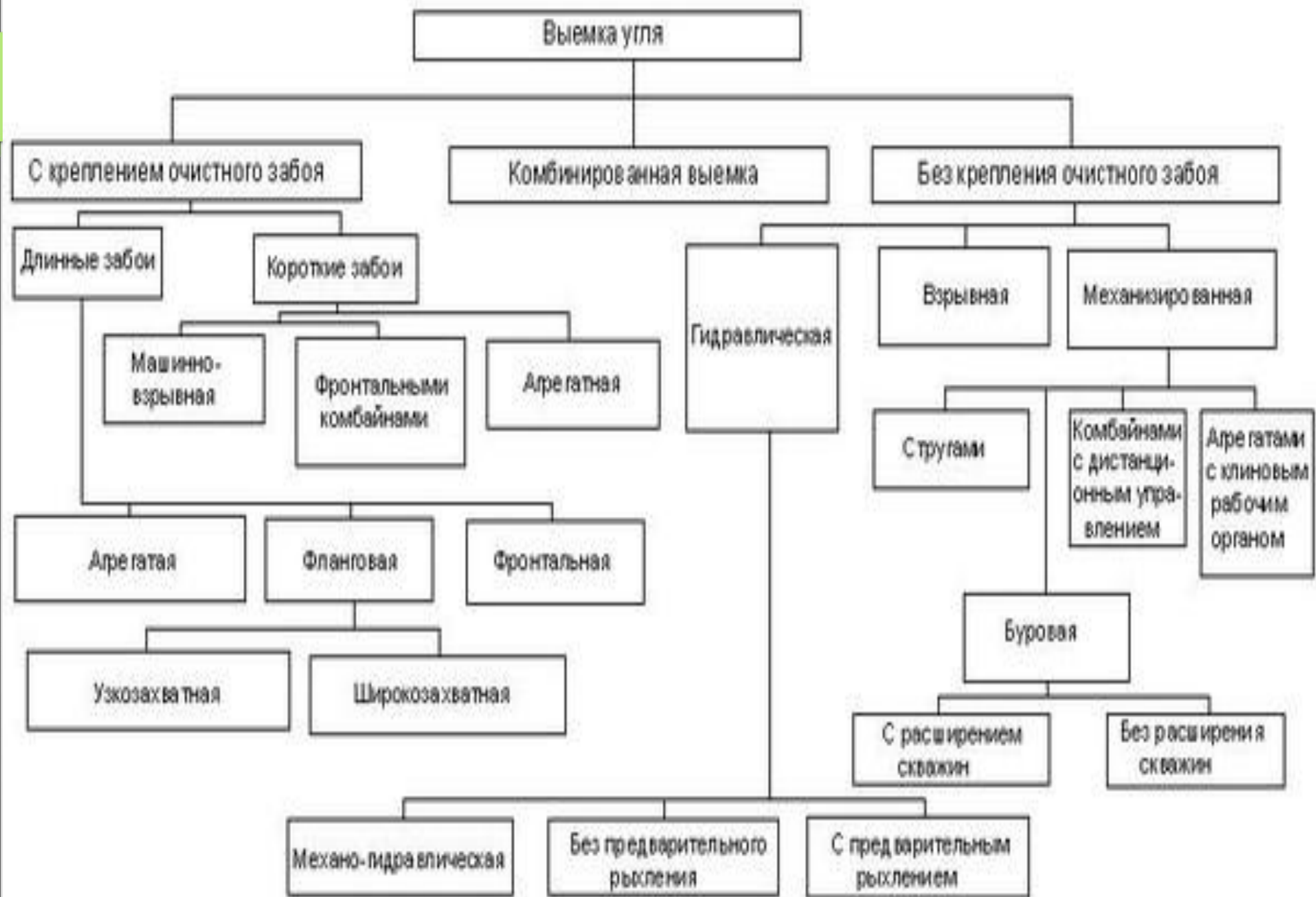
Рис.1. Классификация технологических схем выемки
