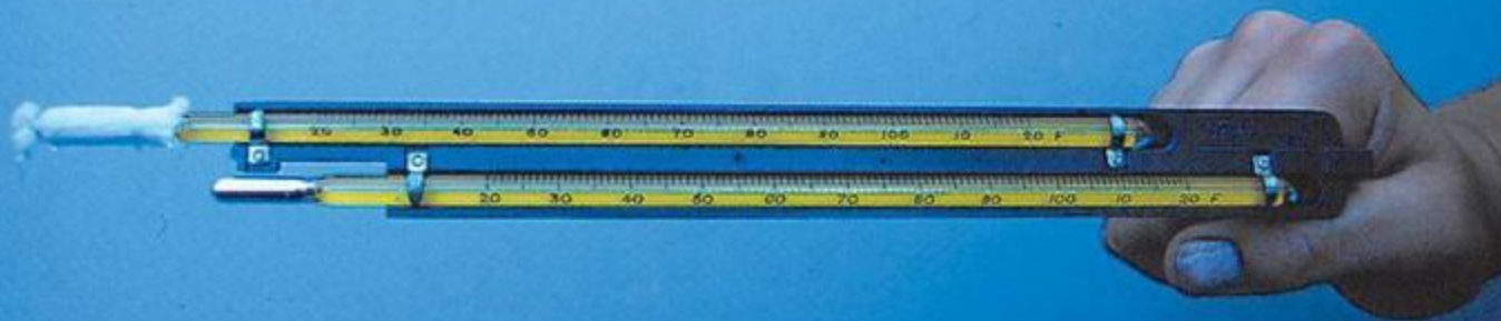
Психрометр
