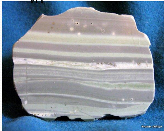
Офиокальцит ит
