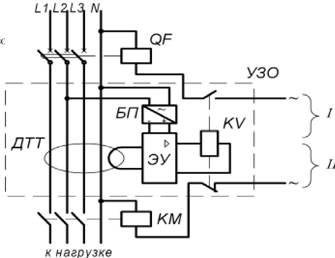
Рисунок – Элементы схемы отдельного электронного УЗО и связь его исполнительного реле KV с автоматическим выключателем QF (I вариант) и электромагнитным пускателем KM (II вариант):
