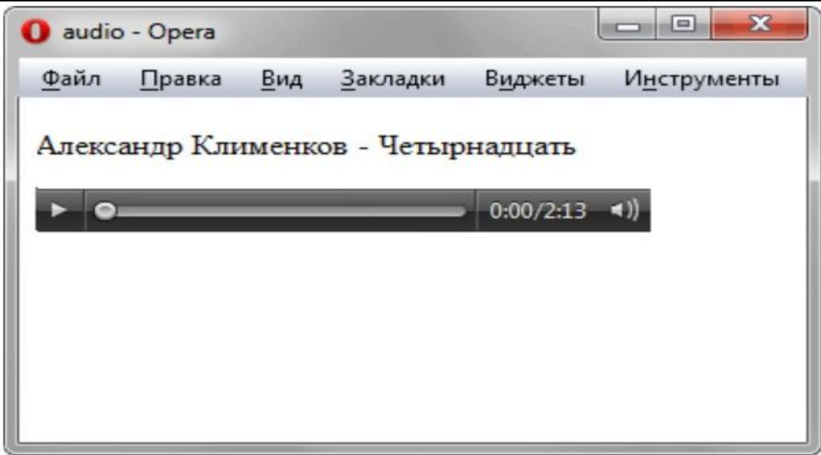
Рис. 1. Воспроизведение аудиофайла
