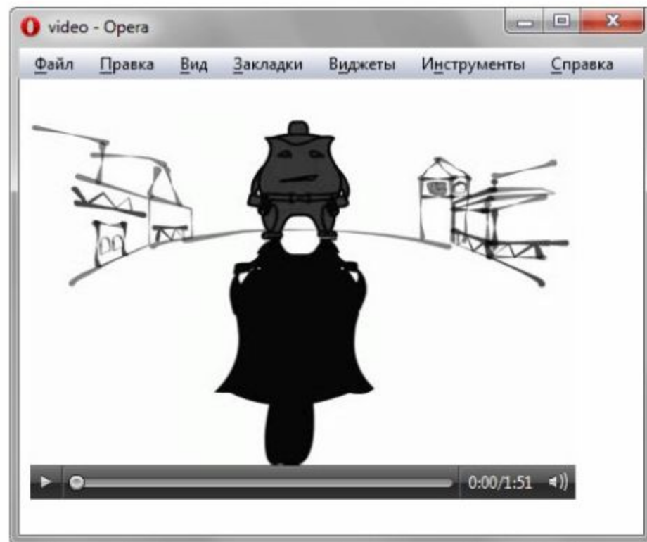
Рис. 1. Воспроизведение видеофайла
