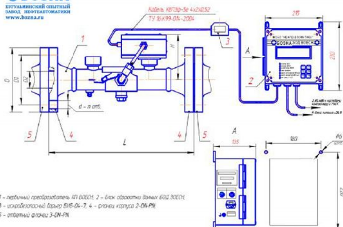
Влагомер сырой нефти ВОЕОН
