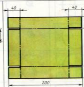
Развертка коробочки
