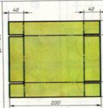
Развертка коробочки
