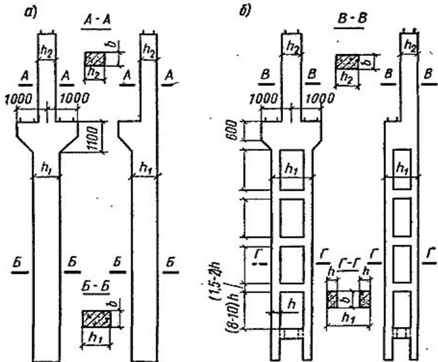
Рис. XIII.9. Колонны одноэтажного здания
