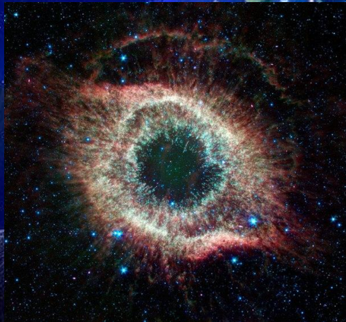
Планетарная туманность Хеликс (Улитка)
