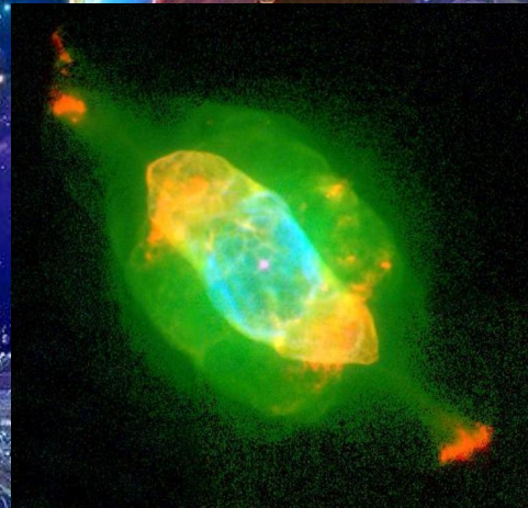
Планетарная туманность Сатурн
